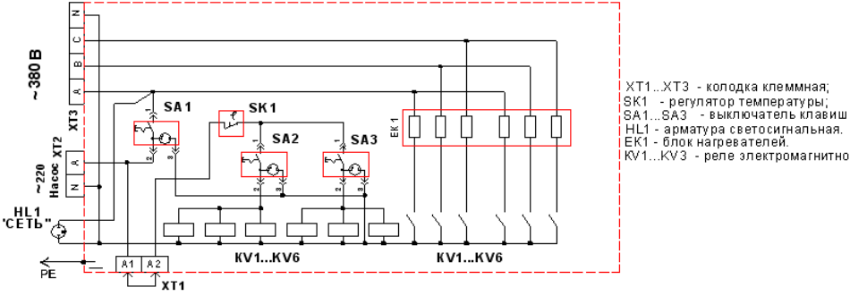
Рис. 5 ЭВПМ-12*...15...18...24 (6 реле, 6 нагревателей)- Схема электрическая принципиальная. ЭВПМ-12* (6 реле, 6 нагревателей) изготавливаются по спец. заказу.
