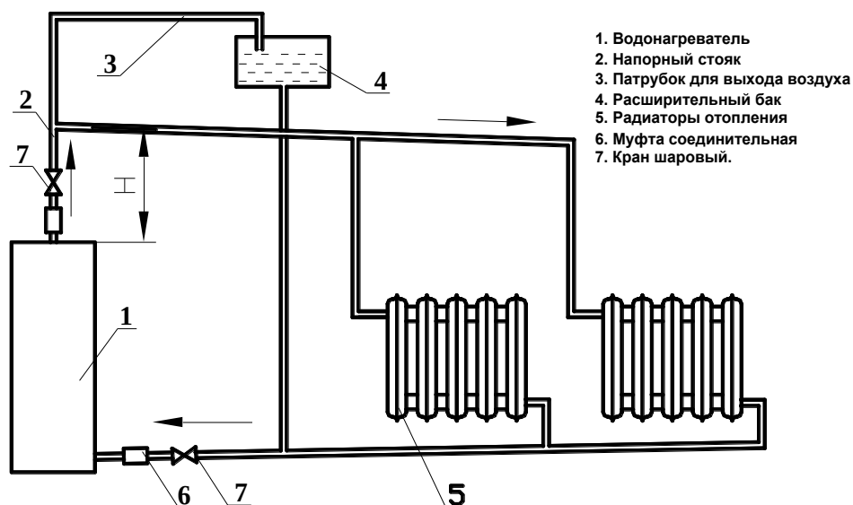
Рис. 6 Схема включения ЭВПМ-12...24 в отопительную систему с естественной циркуляцией.
