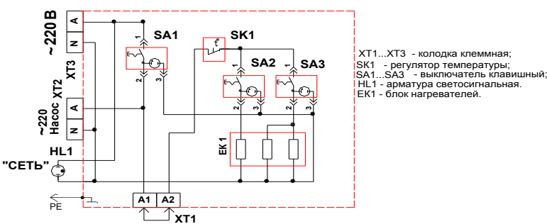
Рис. 2 ЭВПМ-3 Схема электрическая принципиальная.
