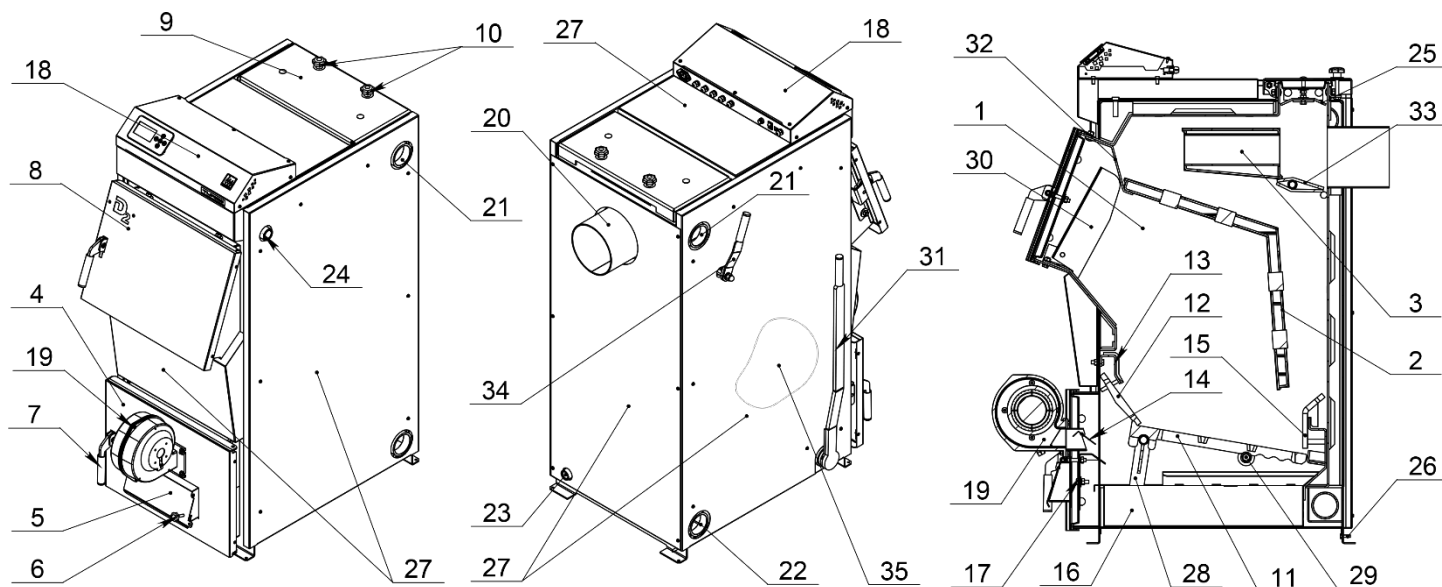
Рис. 2 Устройство котла D2
