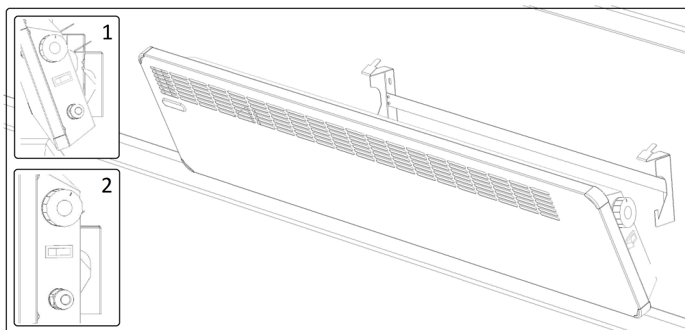
Рис.3 Схема установки
