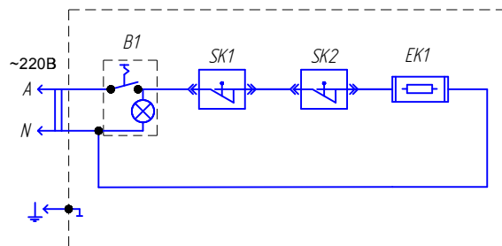
Рис.1 Схема электрическая принципиальная
