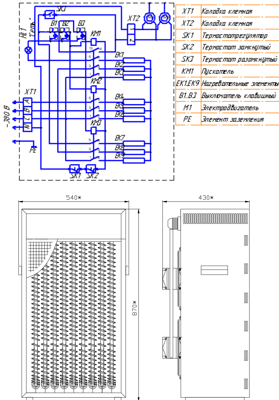
Рис.3. Калорифер КЗВ-42. Габаритный чертеж.
