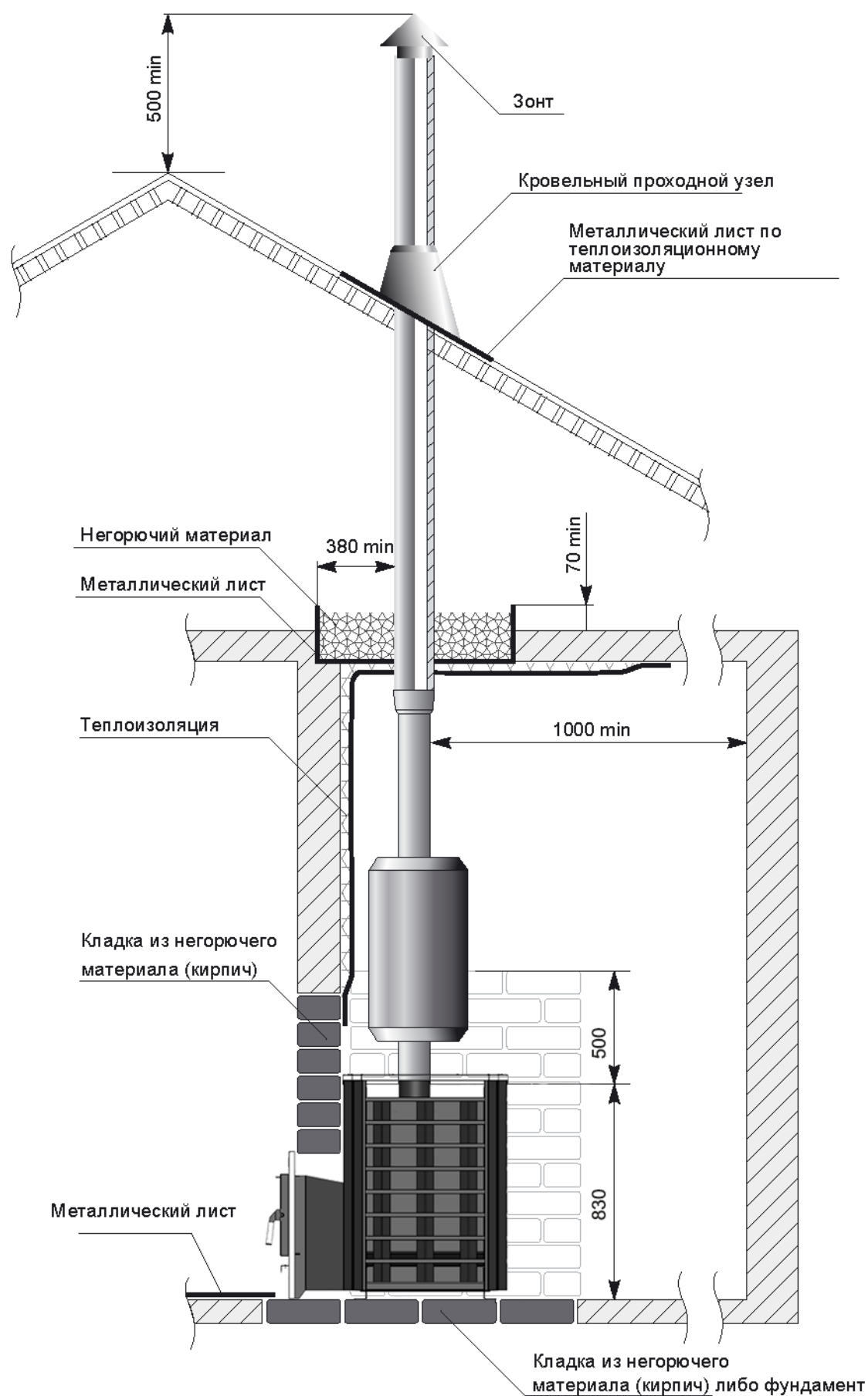
Рис. 4 Схема установки печи BAZALT (вид сбоку)
