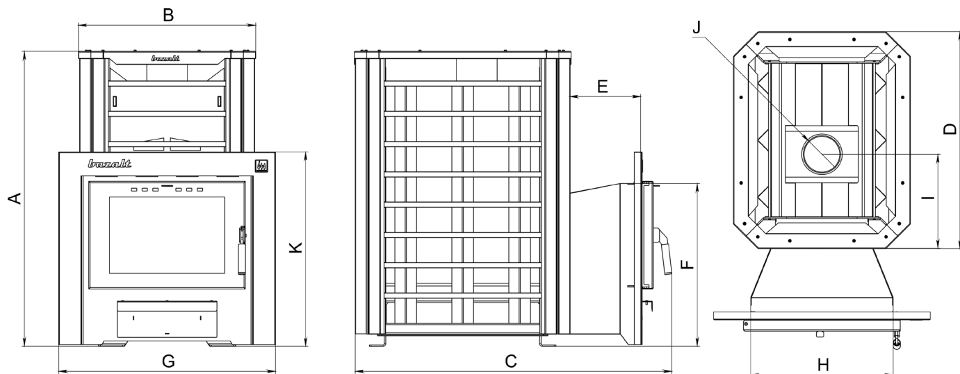
Рис. 2 Основные размеры печи BAZALT
