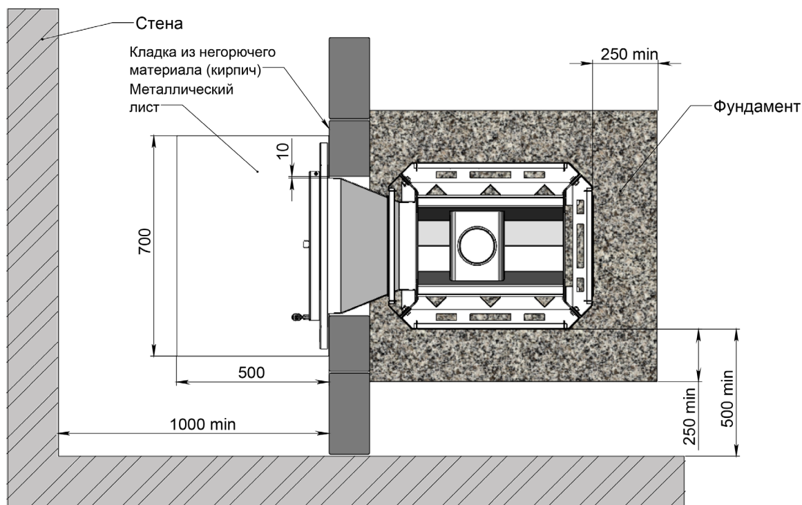
Рис. 3 Схема установки печи BAZALT (вид сверху)
