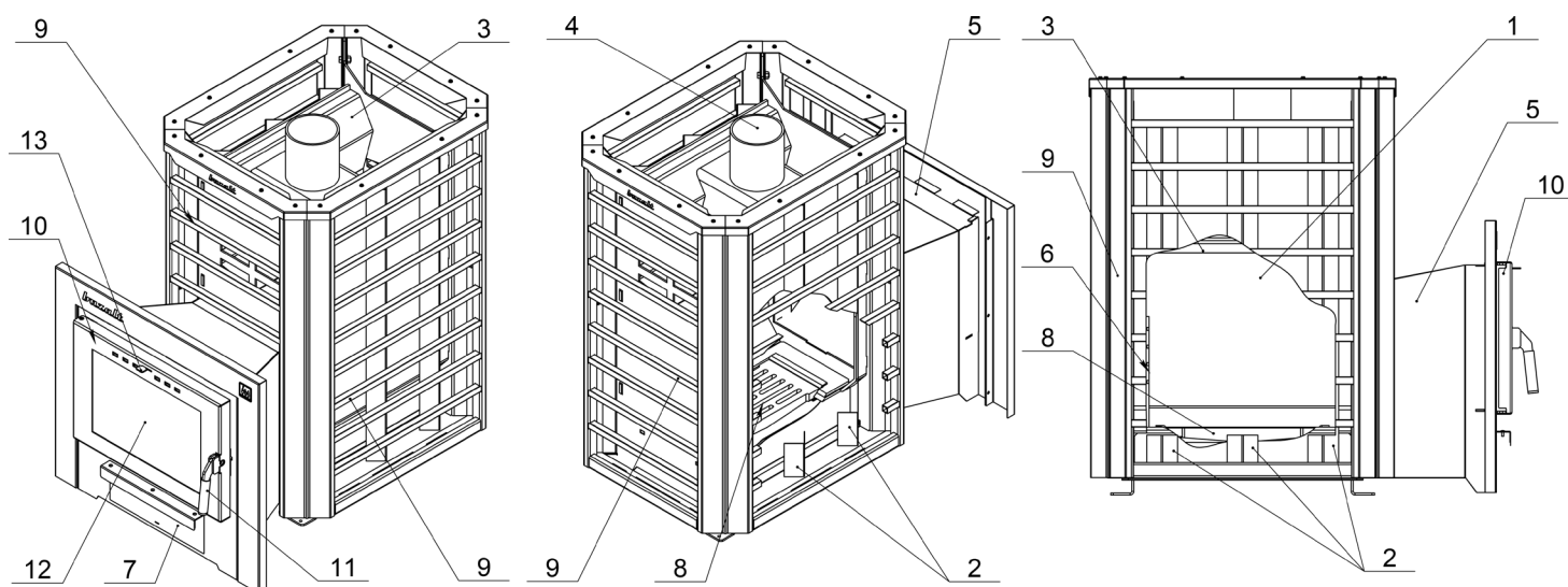
Рис. 1 Устройство печи BAZALT
