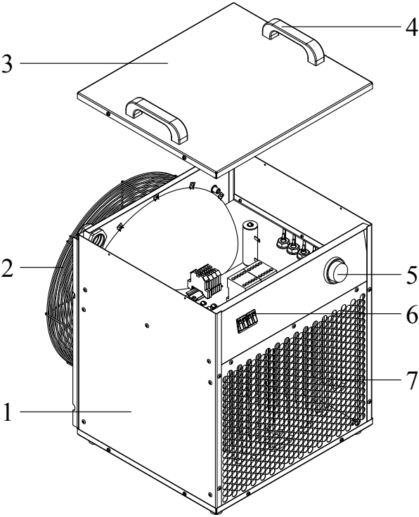
Рисунок 1. Тепловентилятор
