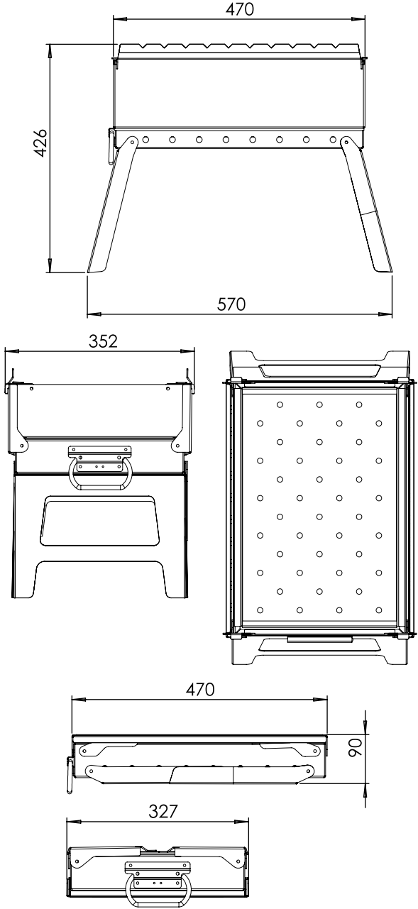
Рис. 1 - Габаритные размеры мангала.
