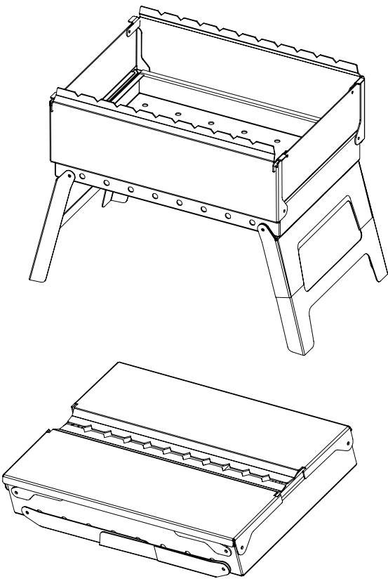
Рис. 2 - Схема мангала в собранном виде и в рабочем состоянии.
