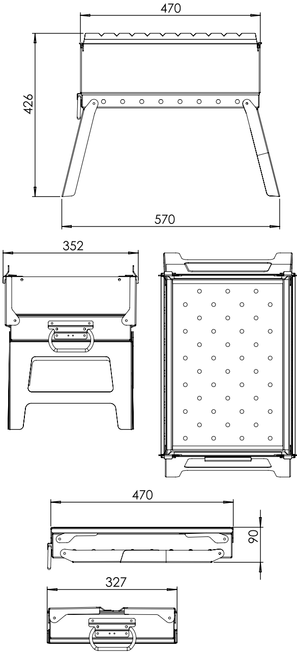
Рис. 1 - Габаритные размеры мангала.
